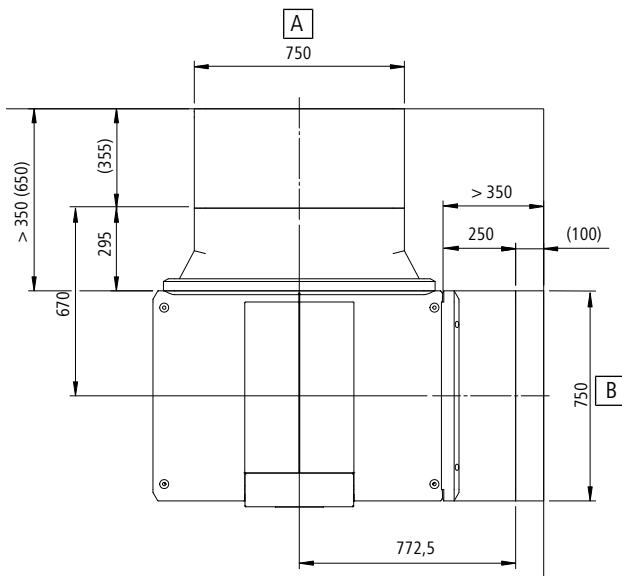
Abb. 6: Abmaße Über-Eck-Montage
