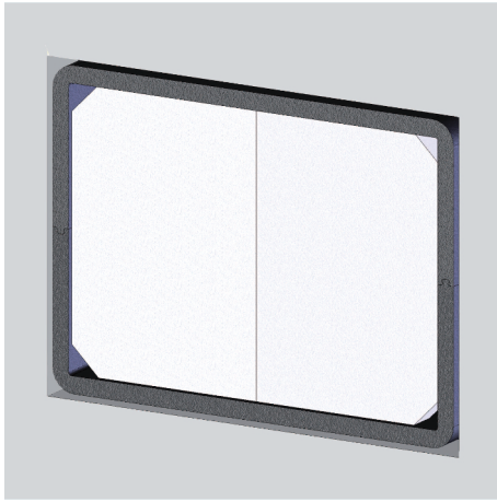
Abb. 16: Spreizplatten anbringen
