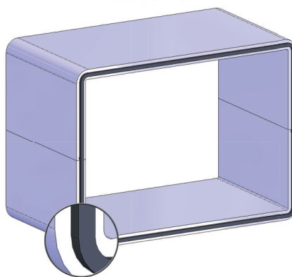
Abb. 14: Kompriband aufkleben
