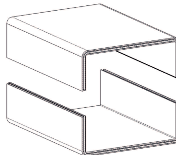
Abb. 5: Halbschalen Luftkanal 90°, W40024
