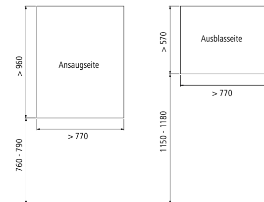
Abb. 8: Mauerdurchbrüche und Abstände
