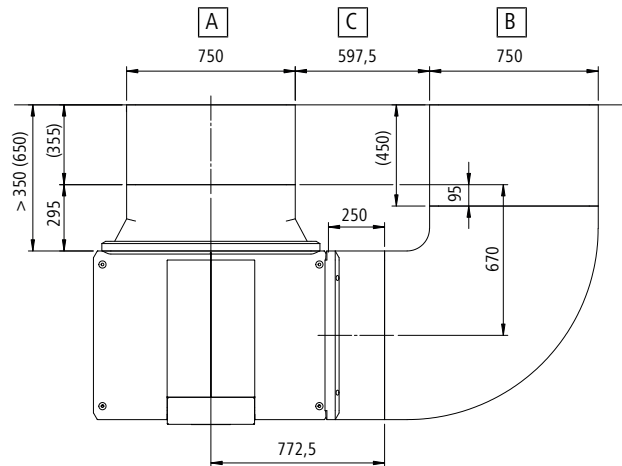
Abb. 7: Abmaße Parallel-Montage
