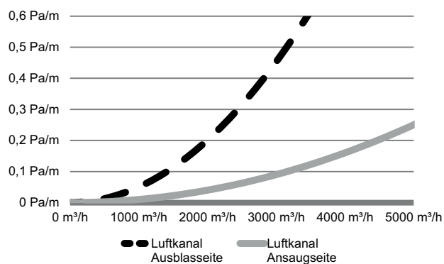
Abb. 18: Druckverlustkennlinie Kanal
