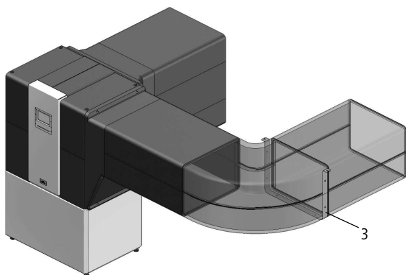
Abb. 13: Haltebügel anbringen
