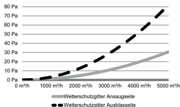
Abb. 20: Druckverlustkennlinie Wetterschutzgitter
