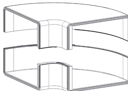
Abb. 5: Halbschalen Luftkanal 90°, W40024
