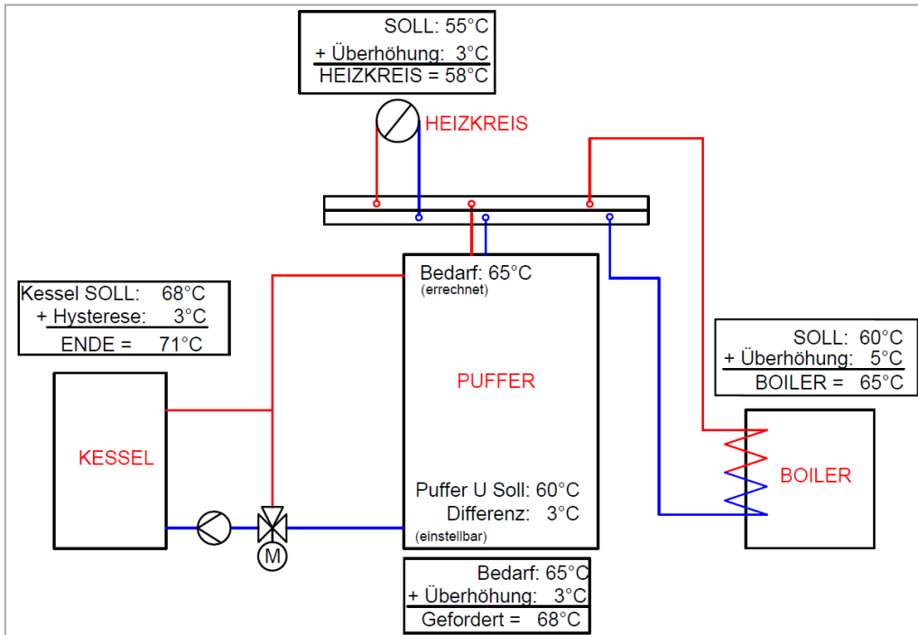
Bild 8.2: Beispiel Temperaturmanager mit Puffer und ohne Differenz
