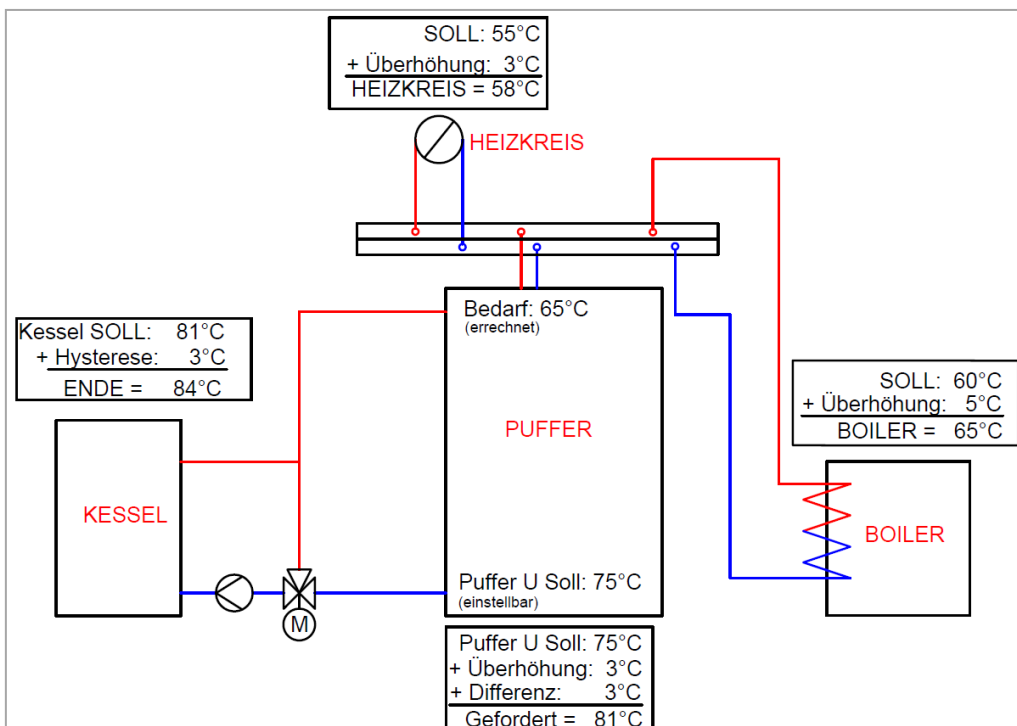
Bild 8.3: Beispiel Temperaturmanager mit Puffer und mit Differenz
