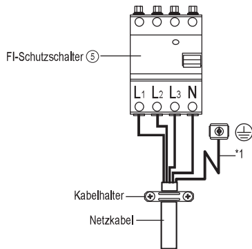
An Klemmen der Trennvorrichtung der Stromversorgung
