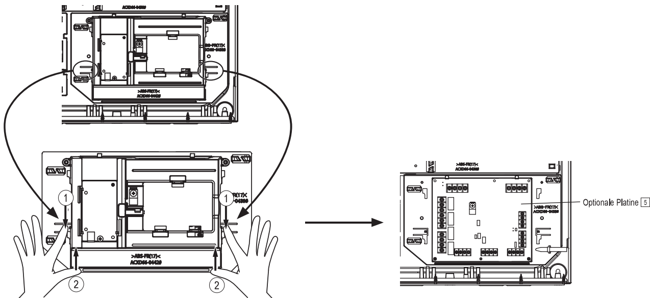
Führung optionaler Kabel- und Netzkabelverbindungen (Ansicht ohne interne Verdrahtung)
