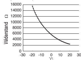
Kennlinie des Speichertemperaturfühlers
