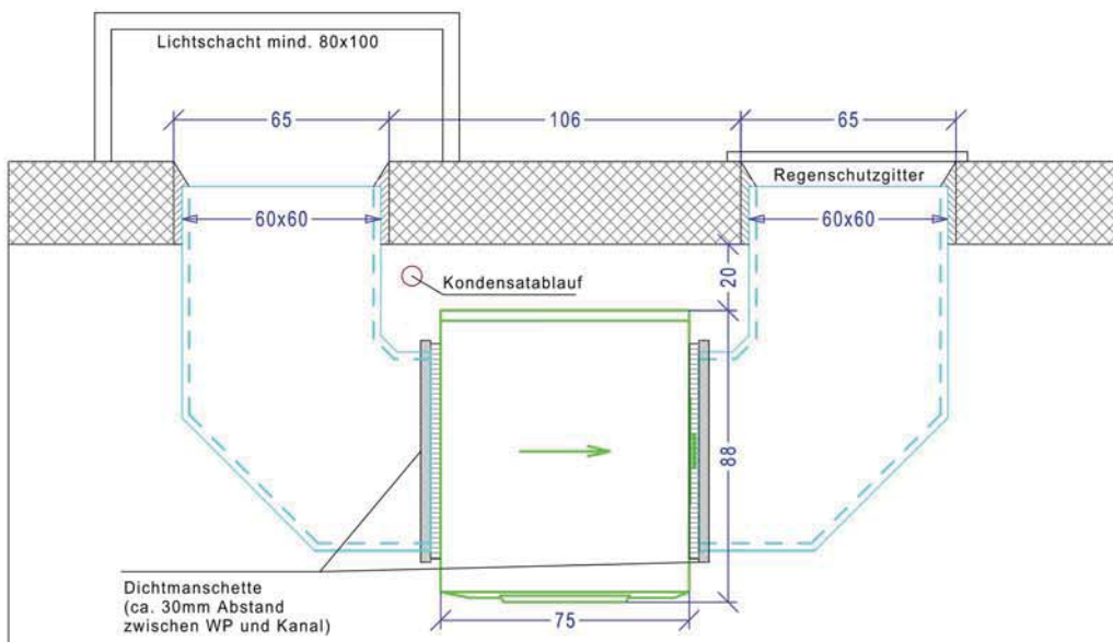
GRUNDRISS (1:25)
